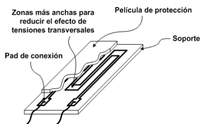
Galga de película metálica
