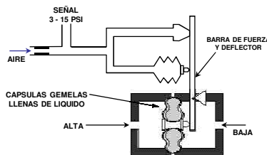
MEDIDORES SECOS
