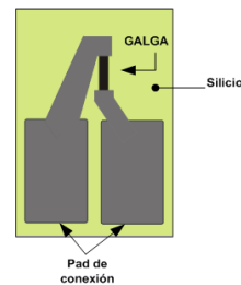
Galgas semiconductoras
