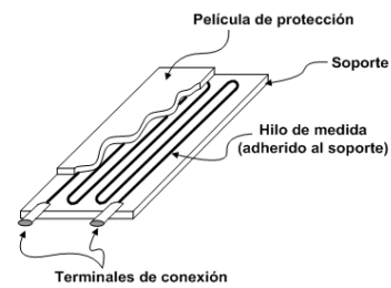
Galga de hilo metálico
