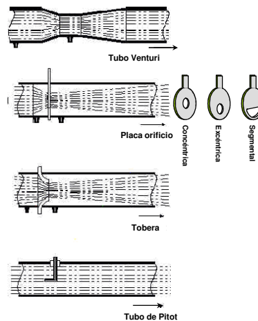
Elementos primarios tipo restricción
